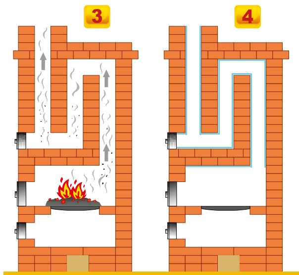
превращение сажи в углекислый газ soot conversion to carbon dioxide
