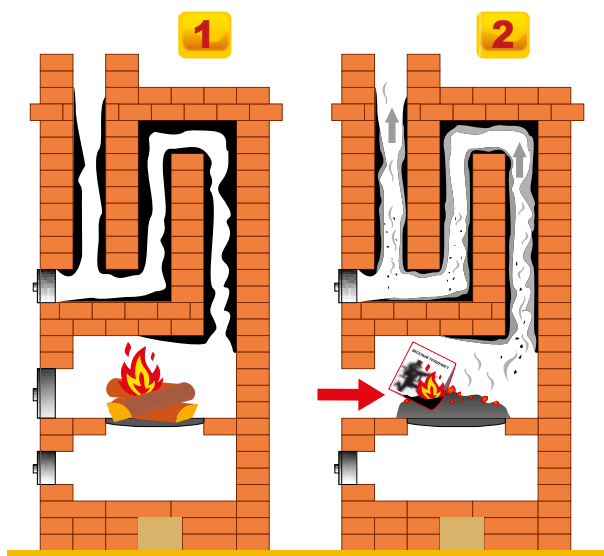
нагрев печи выше 100°C stove heating above 100°C
